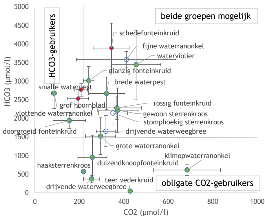
Afbeelding 5. Gemiddelde CO 2 - en HCO 3 - -concentratie in het oppervlaktewater waarbij verschillende submerse beeksoorten voorkomen [1], [2], [3],[ 4], [5]. Lijnen geven de concentraties weer waarboven obligate CO 2 -gebruikers kunnen voorkomen (circa 200 µmol/l CO 2 ), en waarboven er voldoende bicarbonaat is voor bicarbonaatgebruikers om in hun C-behoefte te voorzien (circa 1500 µmol/l HCO 3 - ). Ligt alleen CO 2 boven deze concentratie, dan zijn obligate CO 2 -gebruikers in het voordeel; ligt alleen HCO 3 - boven deze concentratie, dan kunnen alleen bicarbonaatgebruikers voorkomen. Liggen beide concentraties boven deze grenswaarden, dan kunnen beide typen soorten voorkomen, waarbij de obligate CO 2 -gebruikers te maken hebben met concurrentie door HCO 3 - -gebruikers. Groene cirkels betreffen doelsoorten, rode ruiten algemene, woekerende soorten
